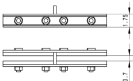
Typ 4: Schienenlasche Hegob, Hassler, VMD
