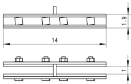
Typ 1: Schienenlasche Lenz alt, Dora 0-Scale
