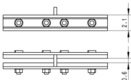
Typ 2: Schienenlasche Lenz neu, Peco Code 143
