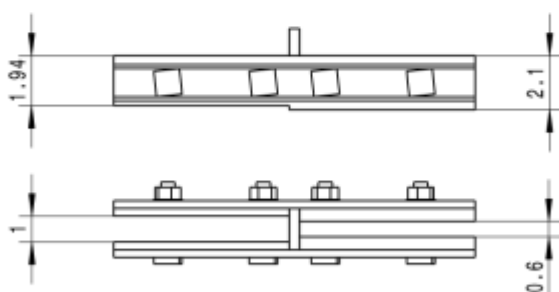
Typ 3: Übergangslasche Lenz alt - neu
